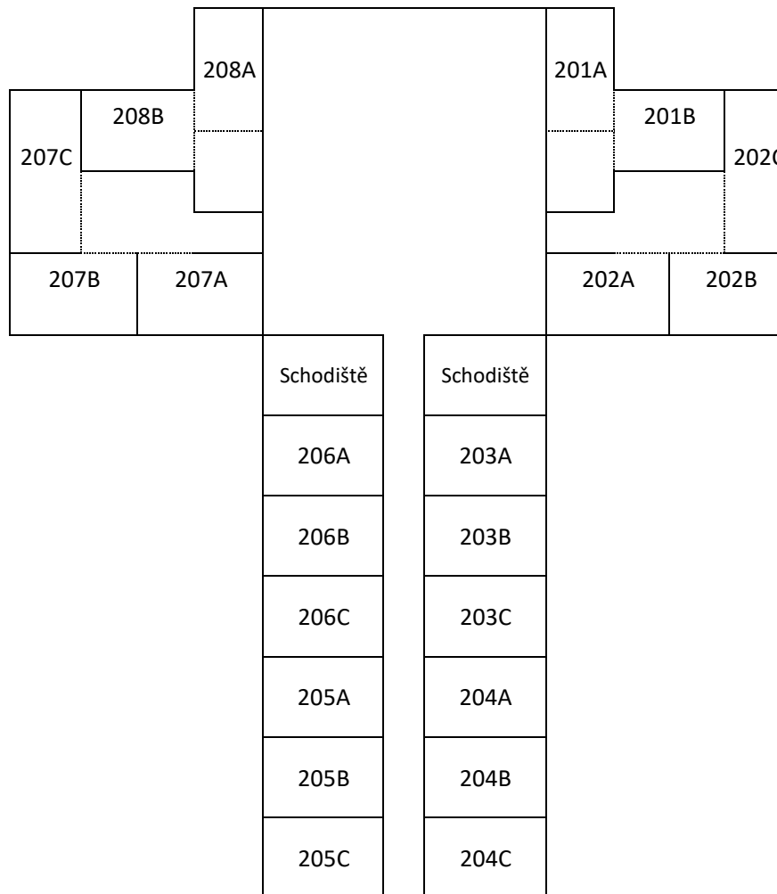
2. nadzemní podlaží
